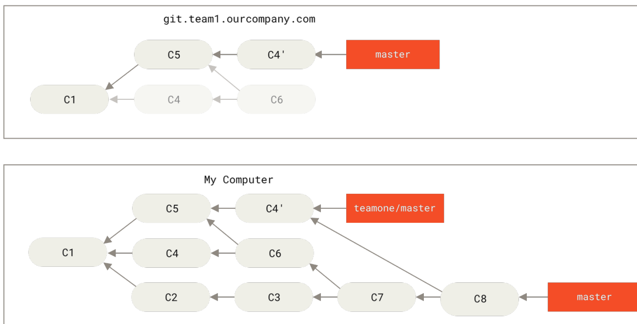
Figure 47. 你将相同的内容又合并了一次，生成了一个新的提交
